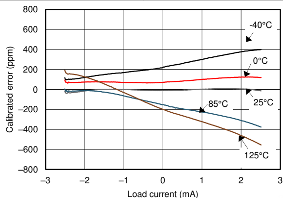
图 10-8. 校准误差与负载电流间的关系
