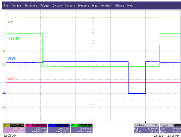
图 9-6. Hardware Reset with /TSMR Press
