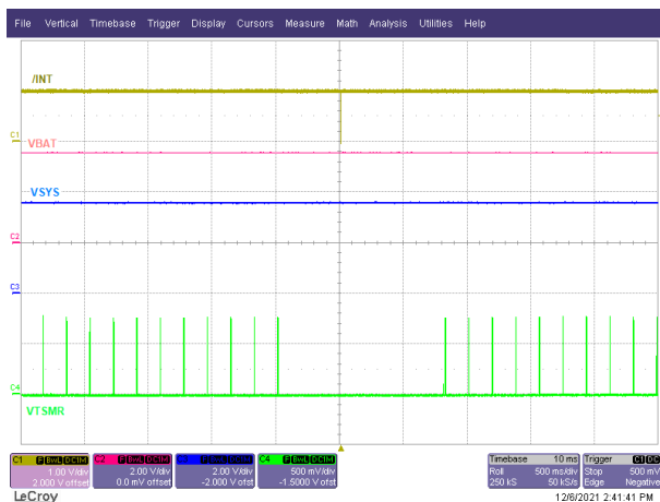
图 9-18. Wake1 Interrupt without VIN
