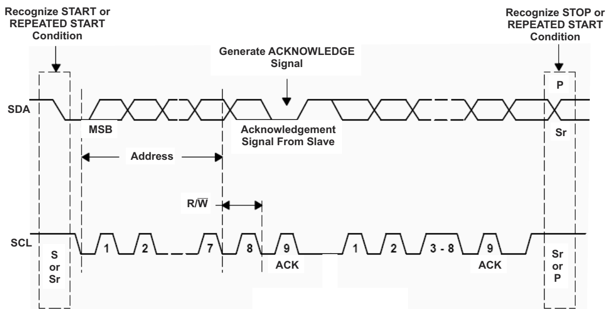
图 8-9. Bus Protocol
