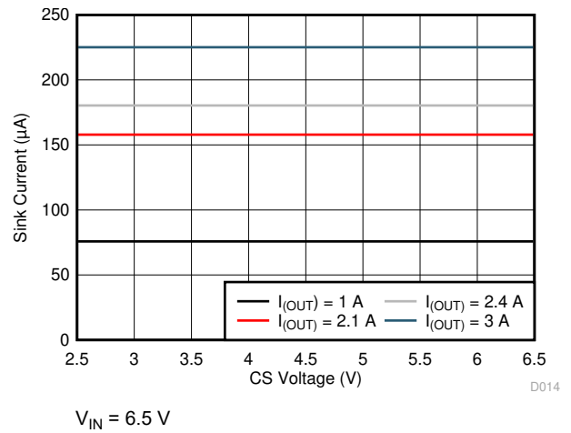
图 6-14. I_{CS} vs V_{CS} Voltage
