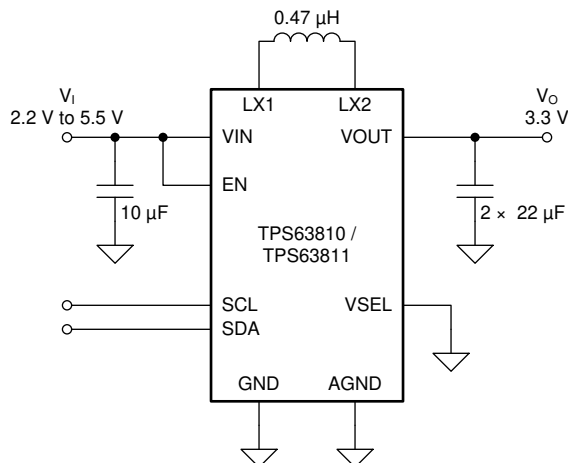
简化原理图
