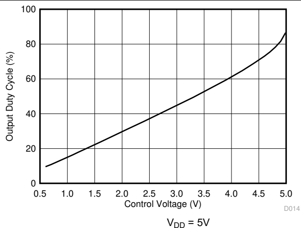
图 7-5. 脉冲位置调制占空比与控制电压间的关系
