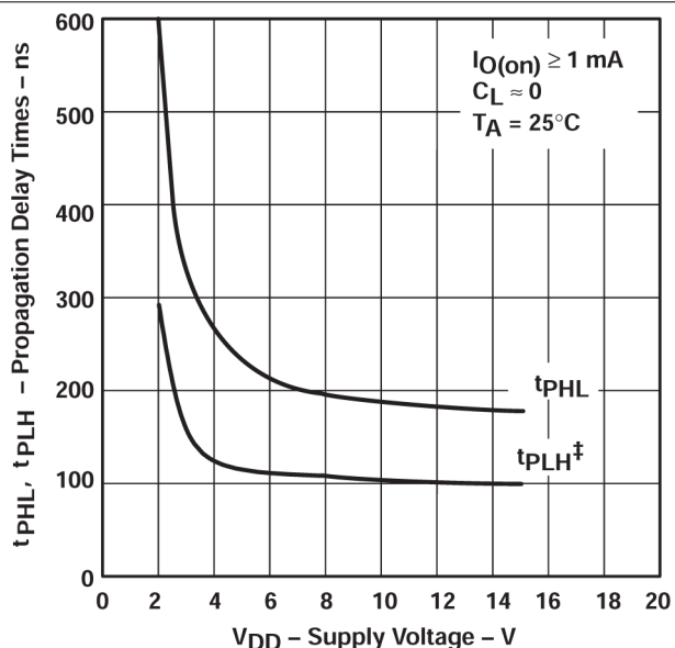
图 5-2. 从触发器到放电输出的传播延迟时间以及和短接阈值与电源电压间的关系
