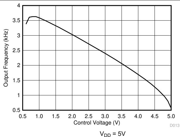
图 7-4. 脉冲位置调制频率与控制电压间的关系
