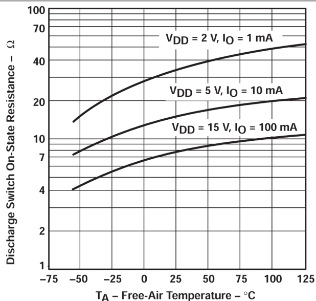
图 5-1. 放电开启状态电阻与自然通风温度间的关系
