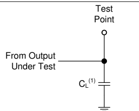
图 5. Load Circuit
