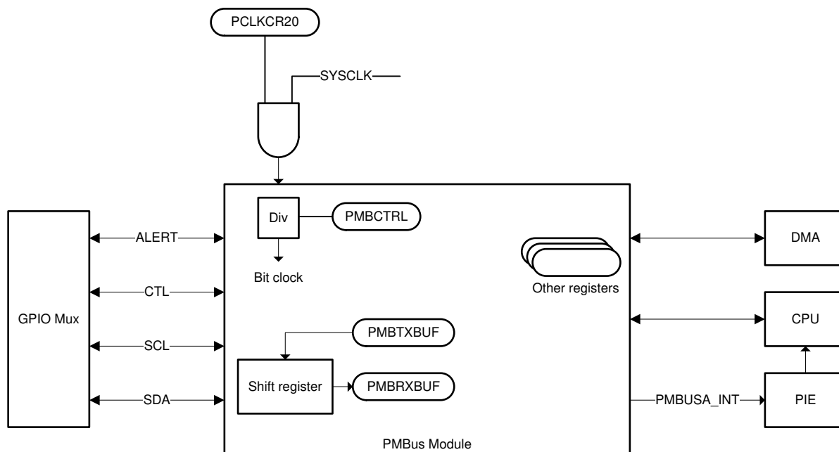
图 6-63. PMBus 方框图
