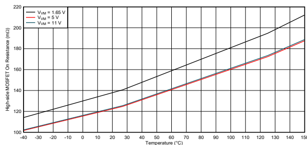
图 7-2. 高侧 MOSFET 导通电阻 (DSG 封装)
