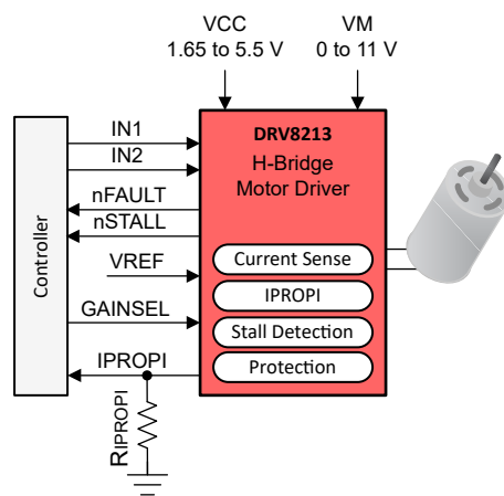
RTE 封装简化版原理图
