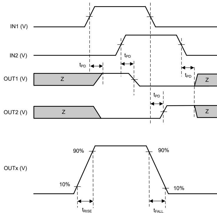
图 7-1. 输入到输出时序
