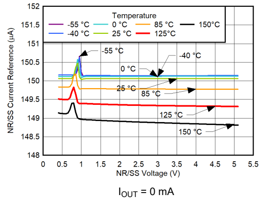
图 6-38. I_{NR/SS} vs V_{NR/SS} and Temperature
