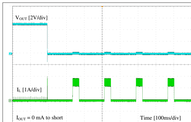
图 8-9. Short Protection
