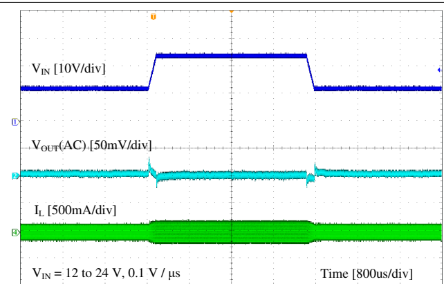
图 8-8. Line Transient
