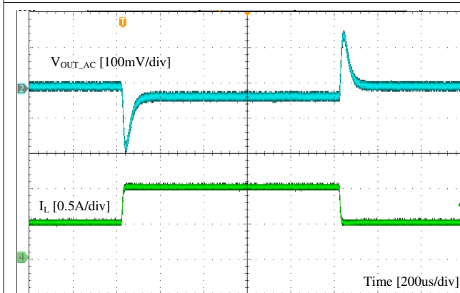
图 8-7. Load Transient
