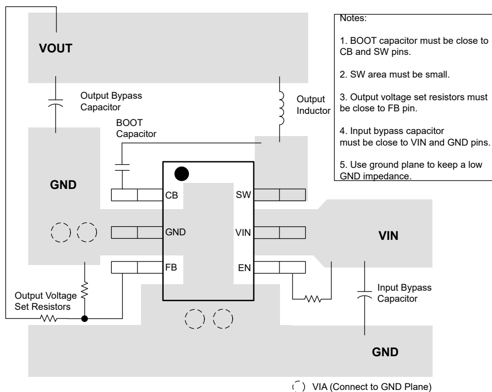
图 8-11. Layout
