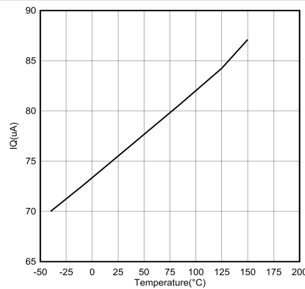
图 6-10. I_Q Versus Temperature
