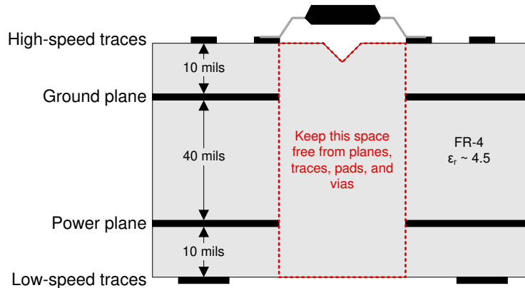
图 8-10. 建议的层堆叠
