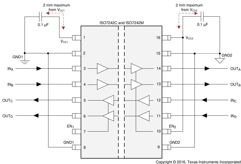
图 8-5. ISO7242x 典型电路组装
