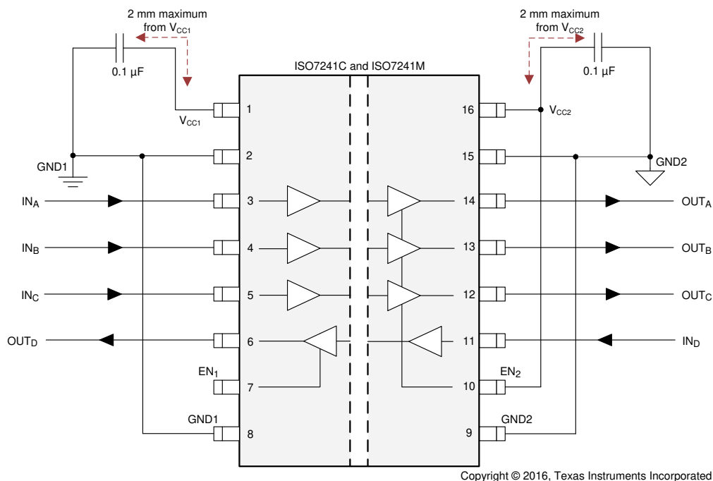
图 8-4. ISO7241x 典型电路组装
