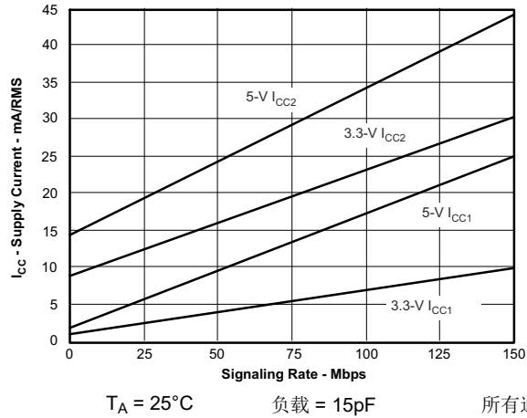
图 5-3. ISO7240C/M RMS 电源电流与信令速率间的关系
