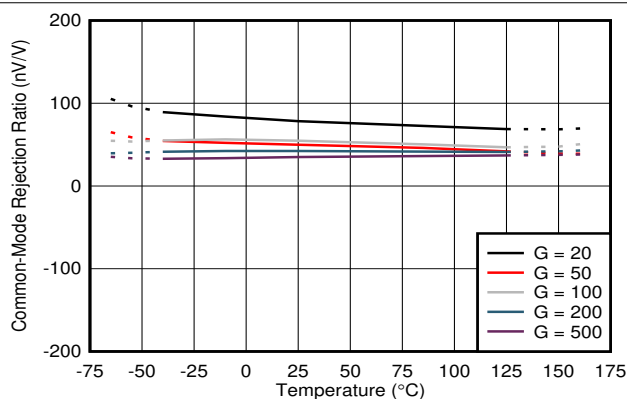
图 5-1. 共模抑制比与温度间的关系
