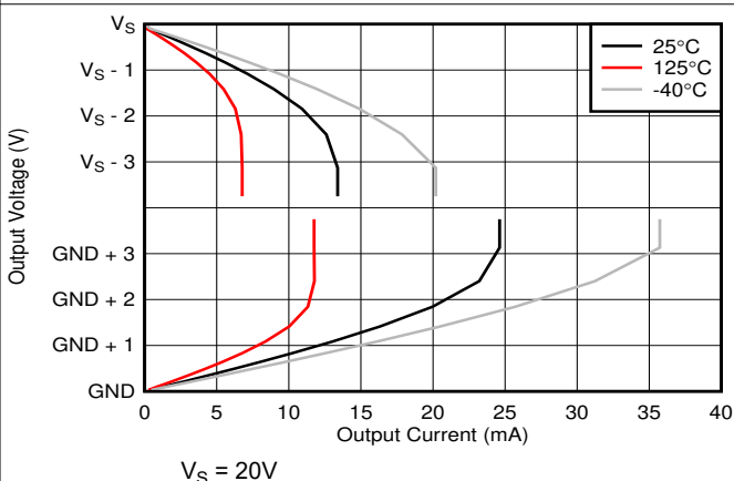
图 5-12. 输出电压与输出电流间的关系
