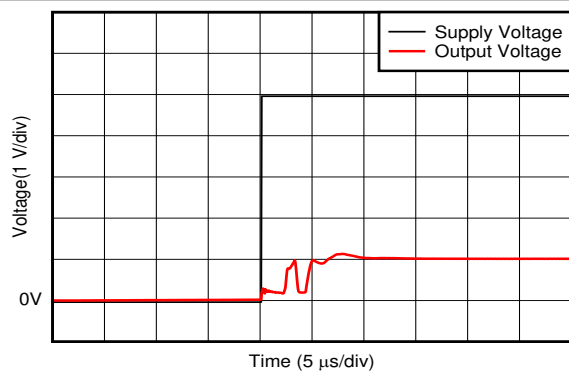
图 5-25. 启动响应
