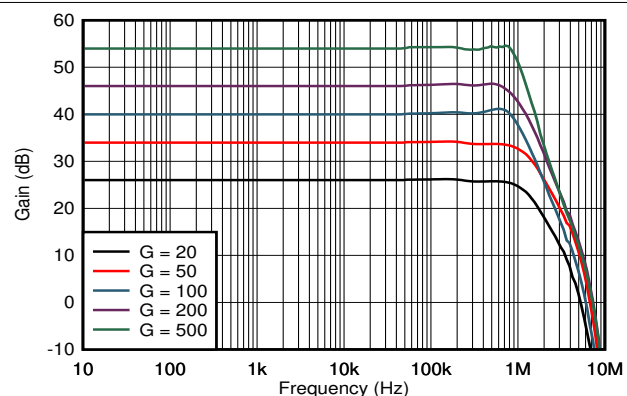
图 5-3. 增益与频率的关系
