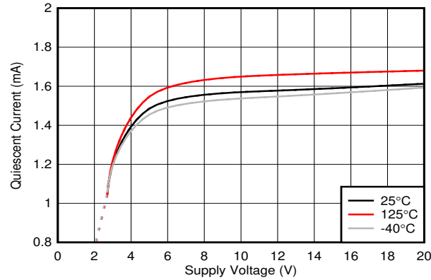
图 5-21. 静态电流与电源电压间的关系
