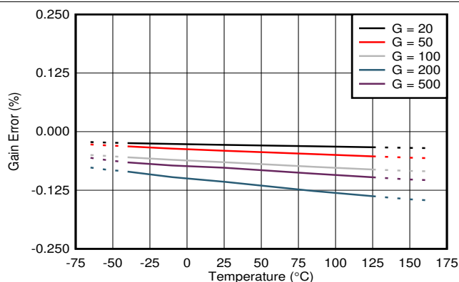
图 5-4. 增益误差与温度间的关系
