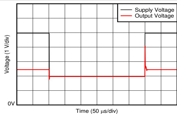
图 5-26. 电源瞬态响应
