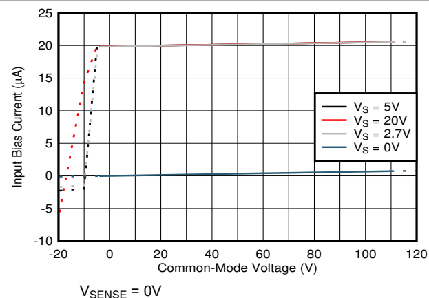
图 5-5. 输入偏置电流与共模电压间的关系
