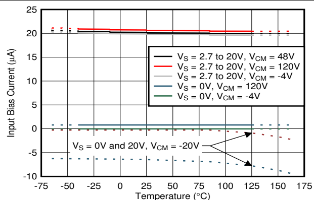
图 5-6. 输入偏置电流与温度间的关系
