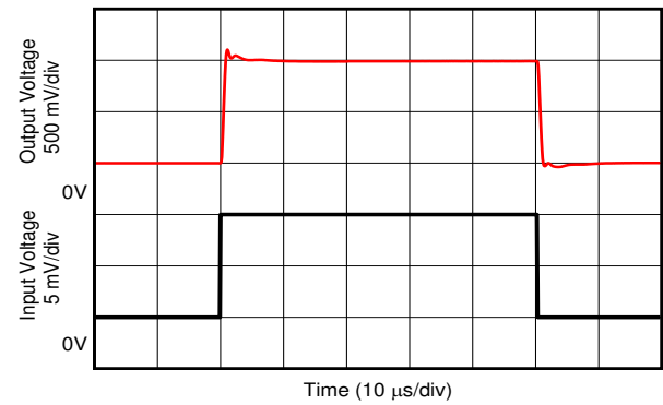
图 5-24. INA281x3 阶跃响应
