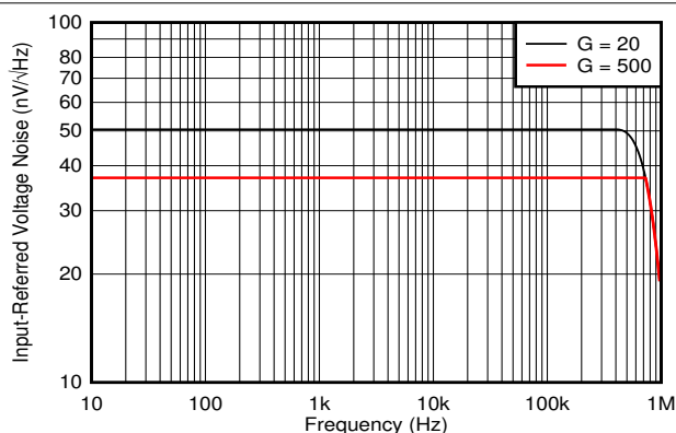
图 5-16. 输入参考噪声与频率间的关系
