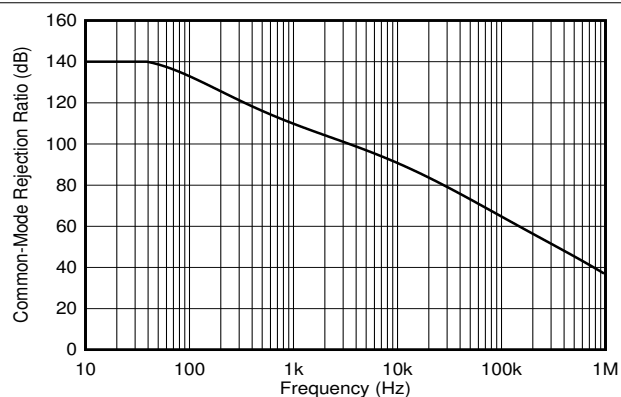
图 5-2. 共模抑制比与频率间的关系
