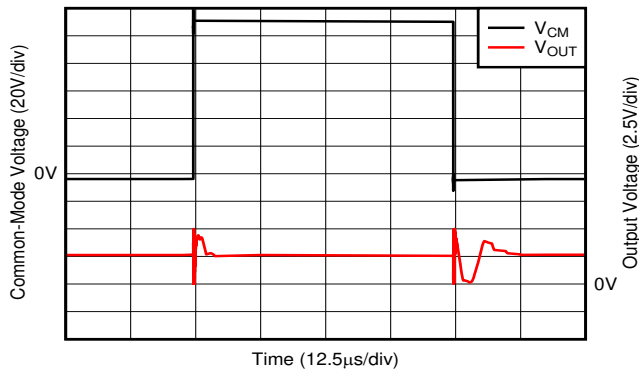
图 5-23. 共模电压快速瞬态脉冲
