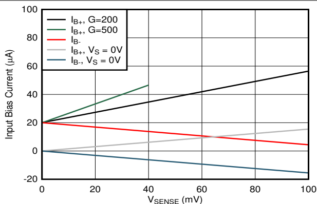
图 5-9. 输入偏置电流与 V_{\text{SENSE}} 间的关系, A4 和 A5 器件
