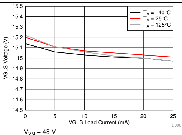
图 7. VGLS Voltage Over Load Current
