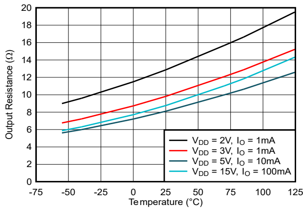
图 5-5. 输出低电阻与温度间的关系
