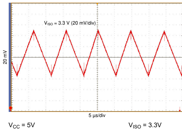
图 7-31. 130 mA 条件下的 V_{ISO} 纹波电压
