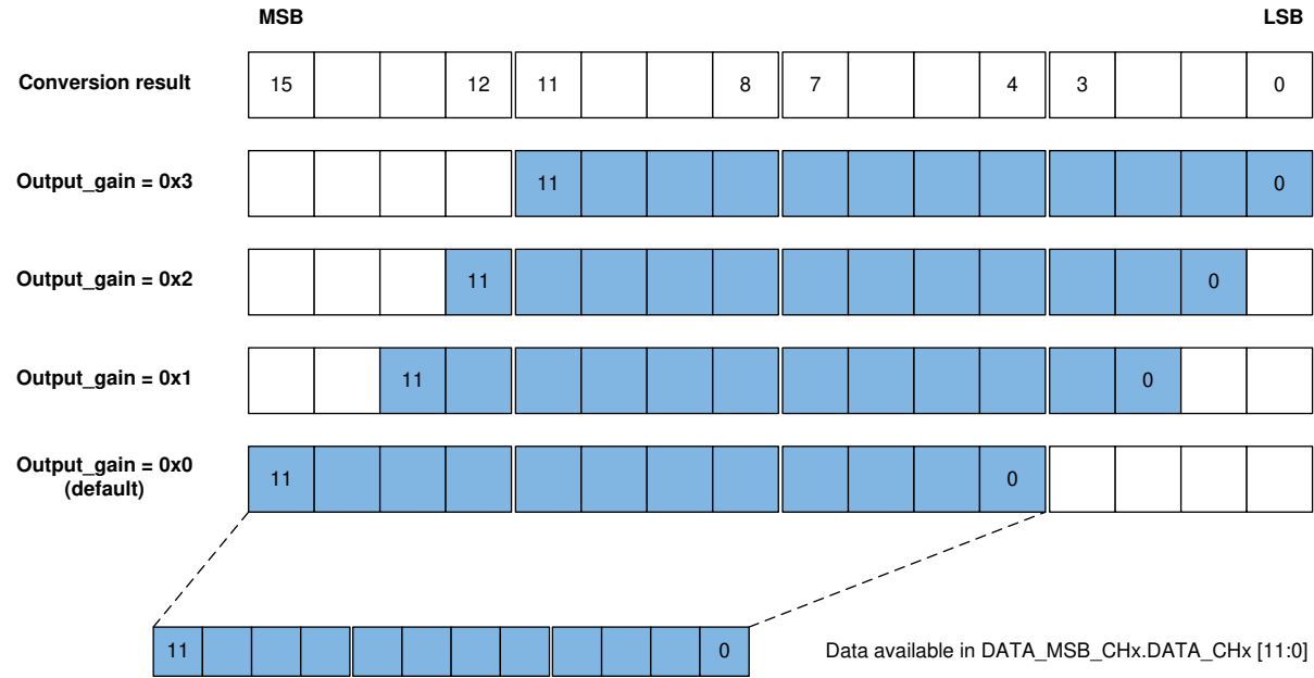
图 7-6. 转换数据输出增益
