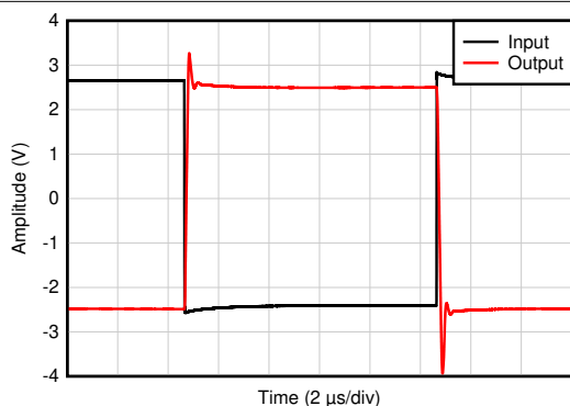
图 5-37. 大信号阶跃响应
