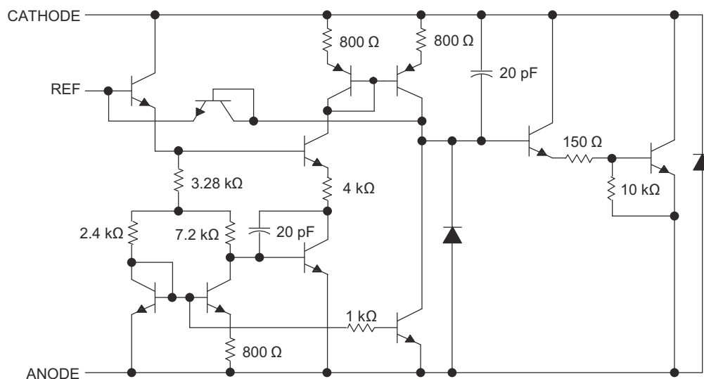
图 8-2. 详细的原理图
