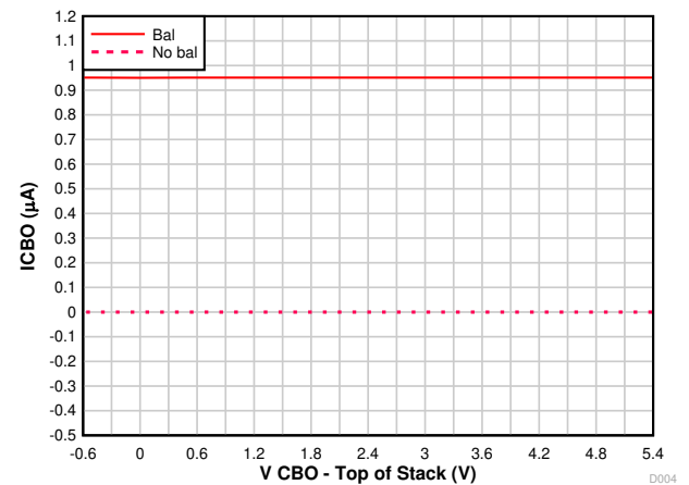
图 8-4. CBO Current Input at 18 V
