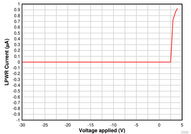
图 8-2. LPWR Current
