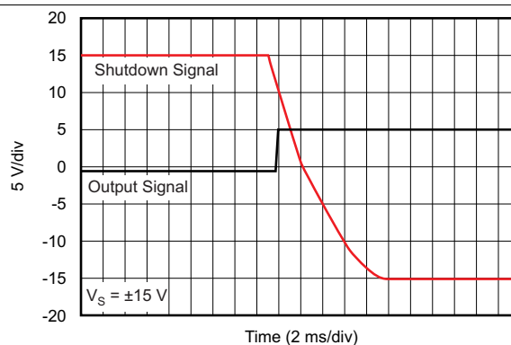
图 38. 无相位反转
