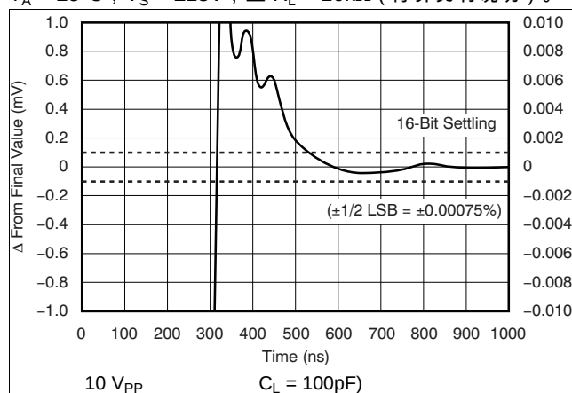
图 31. 大信号正极性建立时间
