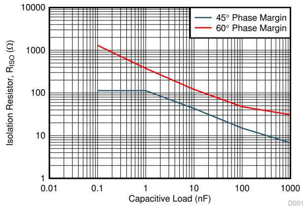
图 7-6. R ISO 与 C LOAD 间的关系
