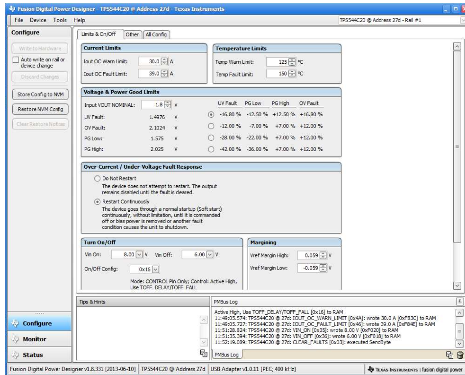
图 49. 使用 Fusion Digital Power Designer 进行器件配置
