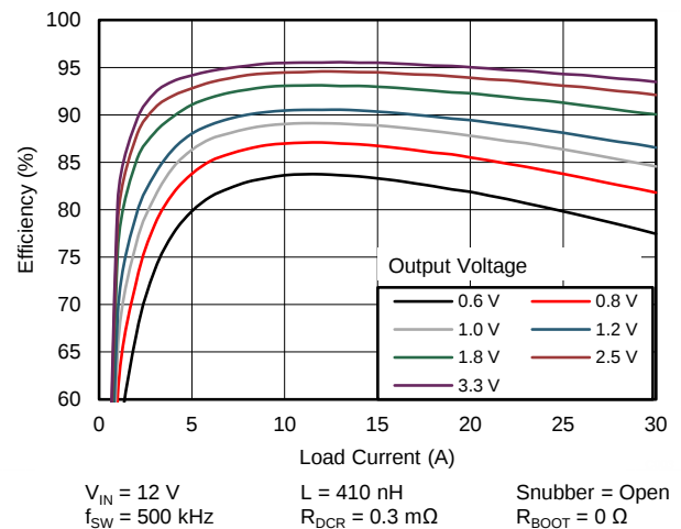
效率与输出电流间的关系
