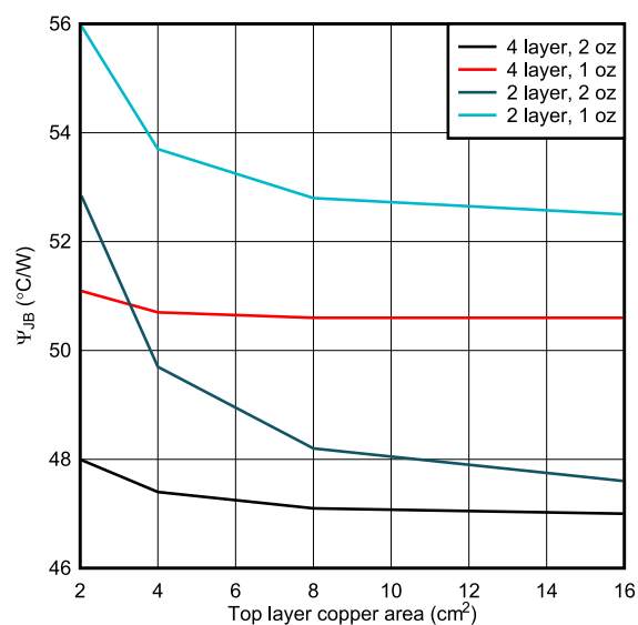
图 9-29. WSON、结至电路板特征参数与铜面积
