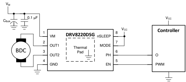
图 9-4. PH/EN 接口电机驱动应用
