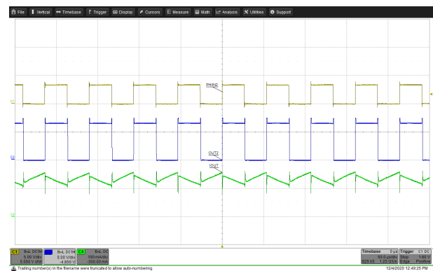
A. 通道 1 = IN2 通道 2 = V_{OUT2} 通道 4 = 电机电流 图 9-13. 使用低侧 FET 在具有 50% 占空比的半桥模式下驱动电机
