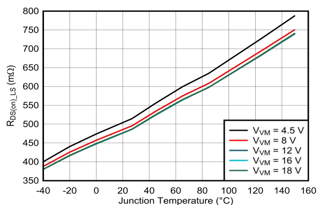
图 7-8. 低侧 R_{DS(on)} 与结温 ( T_J )
