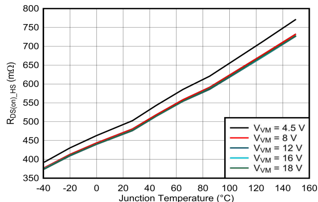
图 7-6. 高侧 R_{DS(on)} 与结温 ( T_J )
