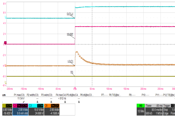
A. 通道 1 = IN1, IN2 (并联) 通道 2 = V_{nSLEEP} 通道 3 = V_{OUT} (OUT1/2 并联) 通道 8 = 电机电流
