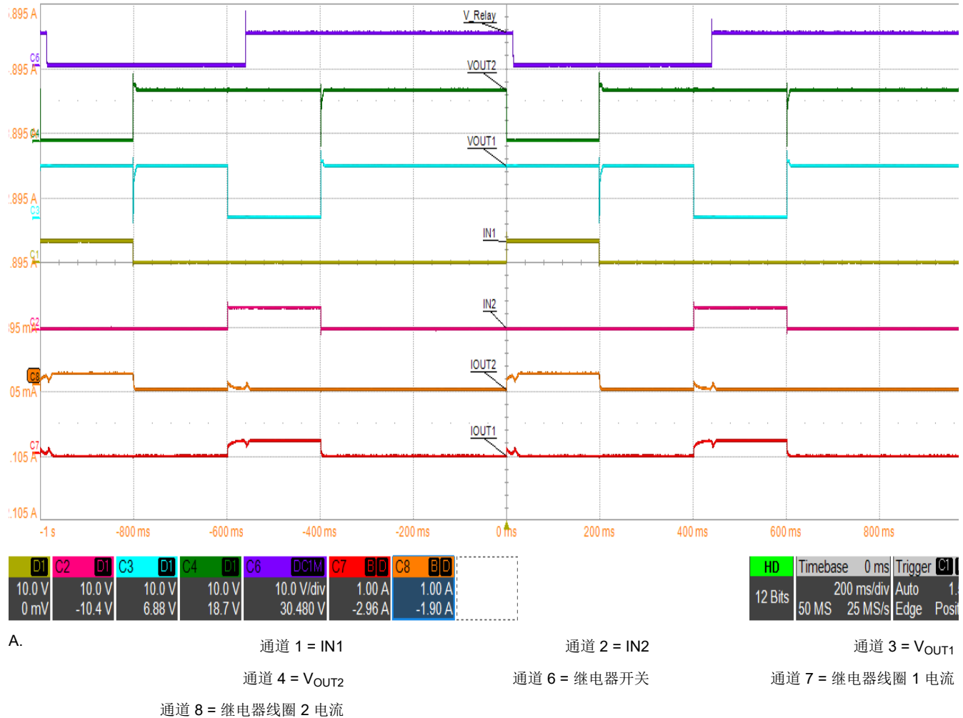
图 9-22. 双线圈继电器的 PWM 驱动
