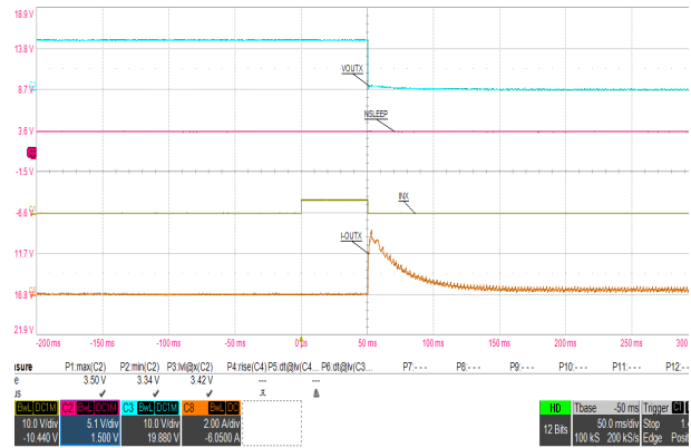
A. 通道 1 = IN1, IN2 (并联) 通道 2 = V_{nSLEEP} 通道 3 = V_{OUT} (OUT1/2 并联) 通道 8 = 电机电流
