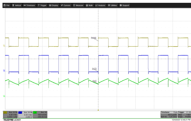
A. 通道 1 = IN2 通道 2 = V_{OUT2} 通道 4 = 电机电流 图 9-12. 使用高侧 FET 在具有 50% 占空比的半桥模式下驱动电机
