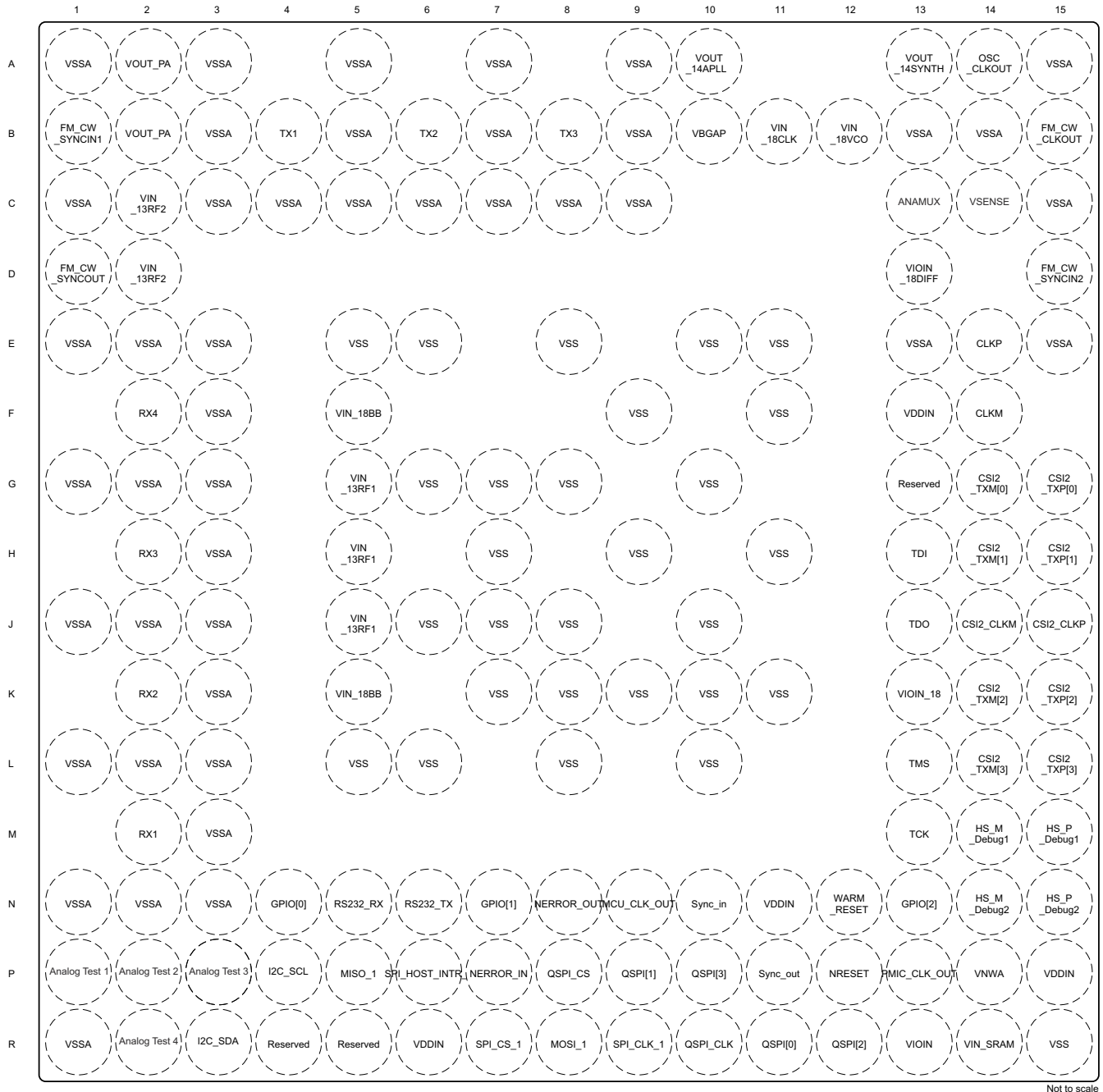
图 6-1. Pin Diagram
