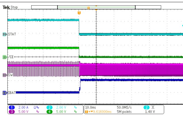
图 10-9. Charge Enable
