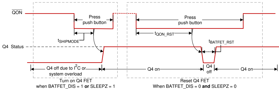
图 9-10. QON Timing
