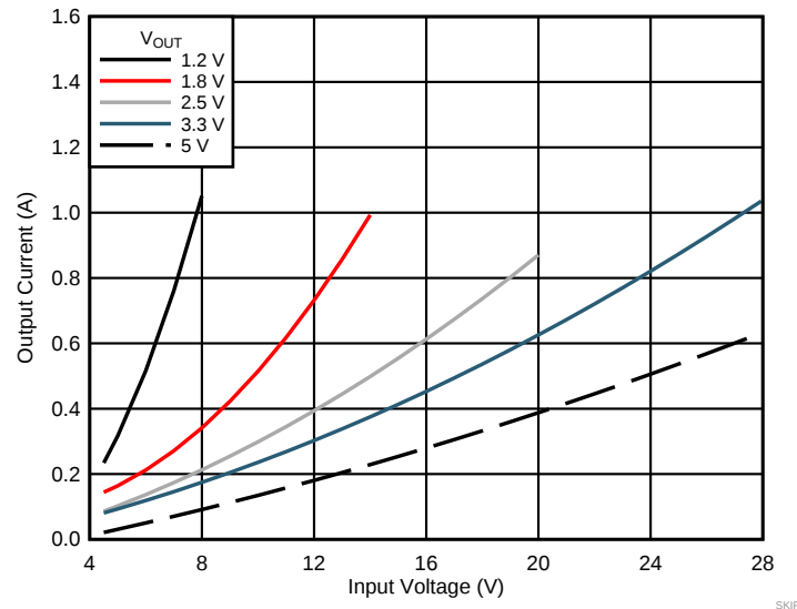
图 26. Pulse-Skipping Threshold
