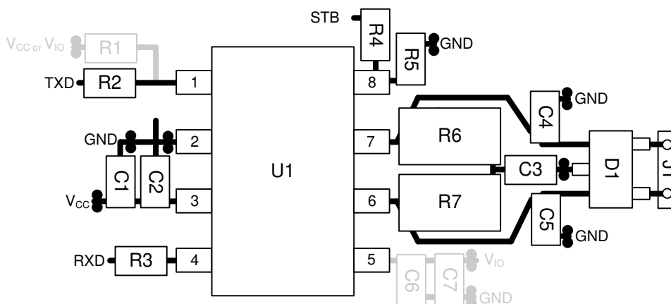
图 12-1. Layout Example
