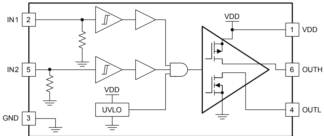
图 36. UCC27538
