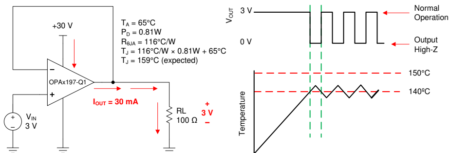
图 7-6. Thermal Protection
