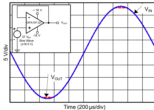
图 6-32. No Phase Reversal
