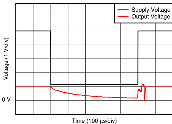
图 6-18. 欠压恢复
