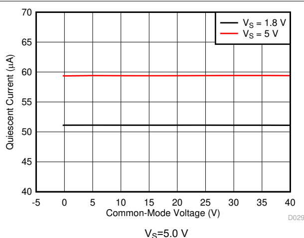
图 6-10. 静态电流与共模电压之间的关系
