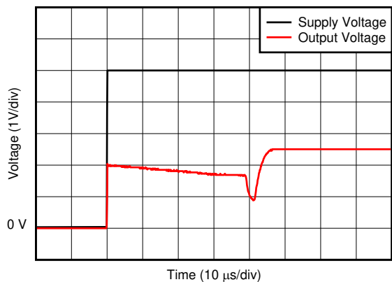
图 6-17. 启动响应
