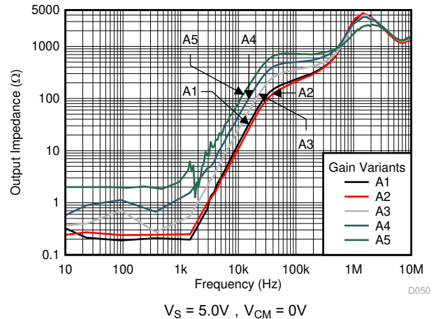
图 6-24. 输出阻抗与频率间的关系
