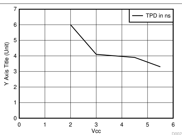
图 5-2. TPD vs V_{CC} at 25^\circ\text{C}
