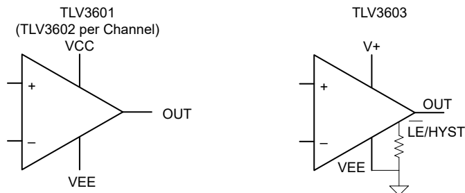
功能方框图
