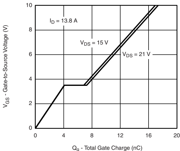
I_D = 13.8\text{ A} V_{DS} = 15\text{ V} V_{DS} = 21\text{ V} Gate Charge
