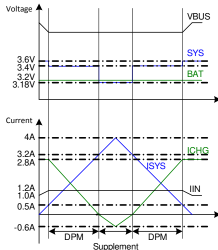
图 9-3. DPM Response
