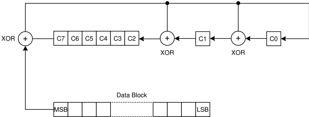
图 8-19. CRC 模块
