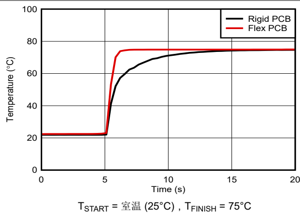
图 7-11. 响应时间
