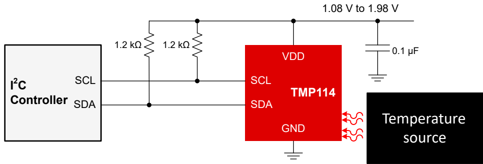
图 9-3. 相同的 I 2 C 上拉和电源电压应用
