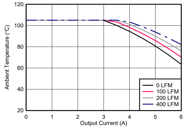
图 7-17. 安全工作区 ( V_{OUT} = 3.3V , F_{SW} = 750\text{kHz} )
