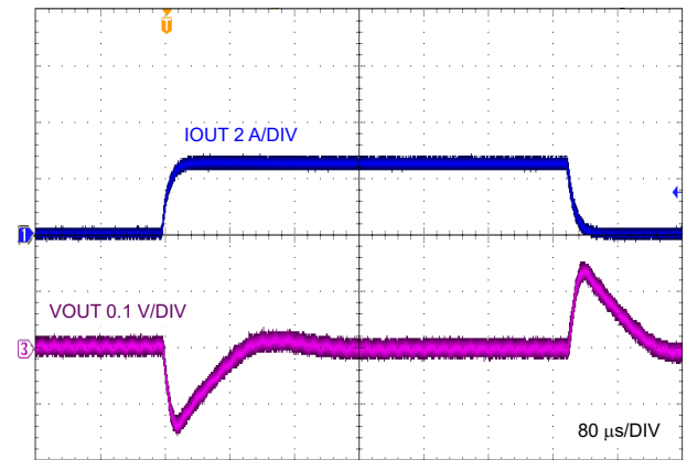
图 9-16. 负载瞬态, 0A 至 2.5A
