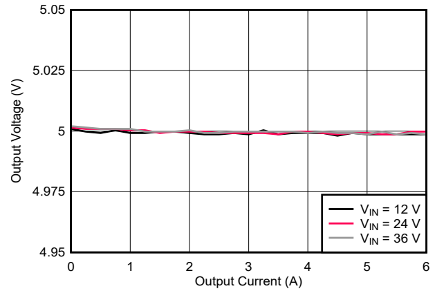
图 9-3. 负载调整率
