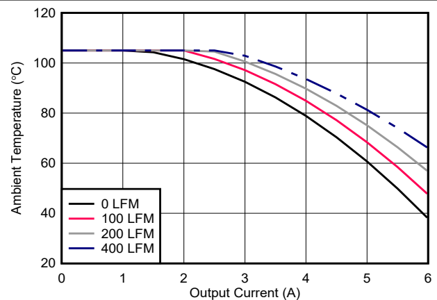
图 7-19. 安全工作区 ( V_{OUT} = 12V , F_{SW} = 2\text{MHz} )
