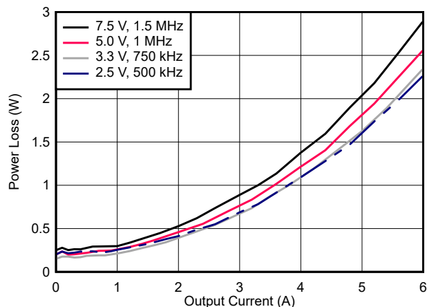
图 7-10. 功率损耗
