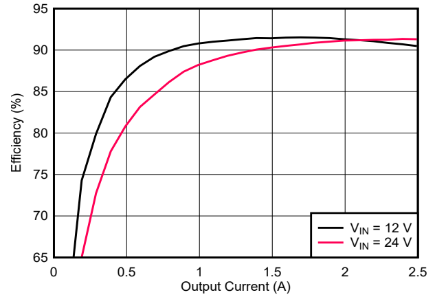
图 9-14. 效率
