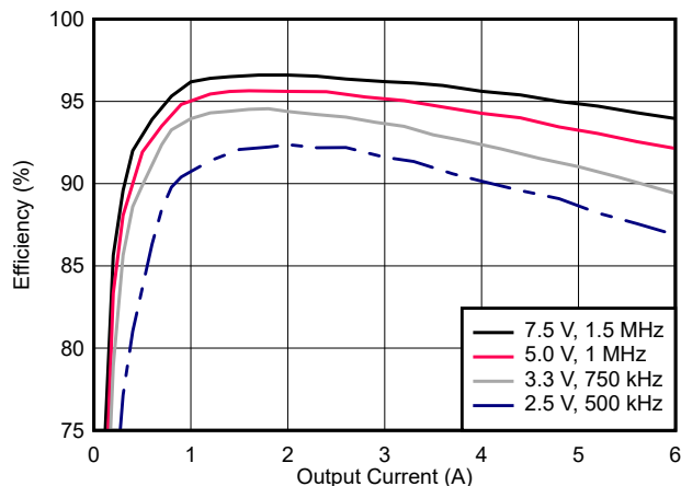
图 7-9. 效率
