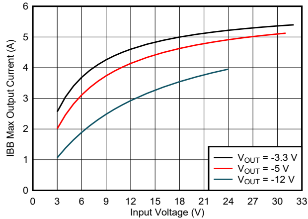
图 9-13. IBB 最大输出电流
