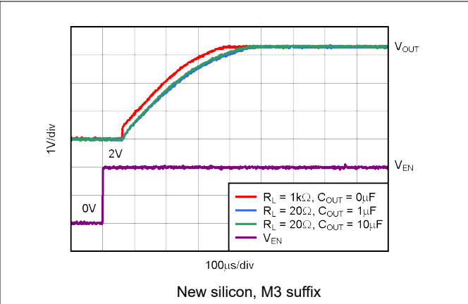
图 7-4. TPS73233 Turn-On Response
