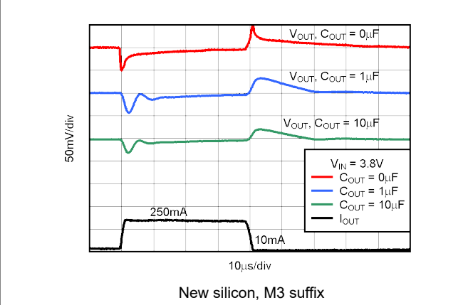
图 7-6. TPS73233 Load Transient Response
