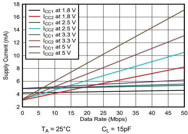
图 6-3. ISO6760L 电源电流与数据速率间的关系 (具有 15pF 负载)
