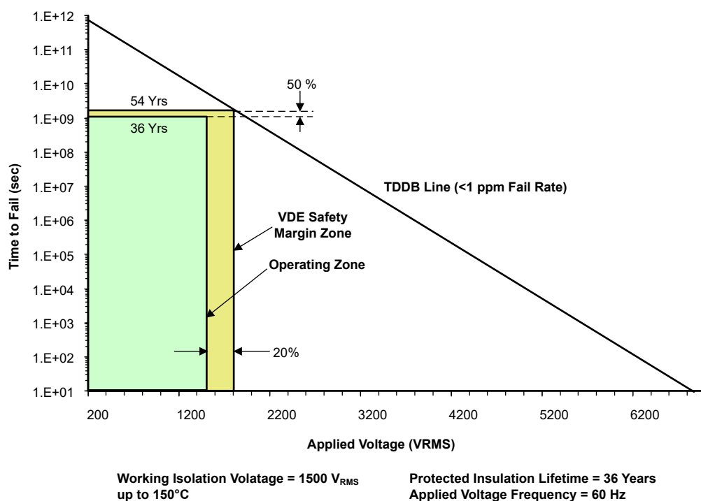
图 10-2. 绝缘寿命预测数据
