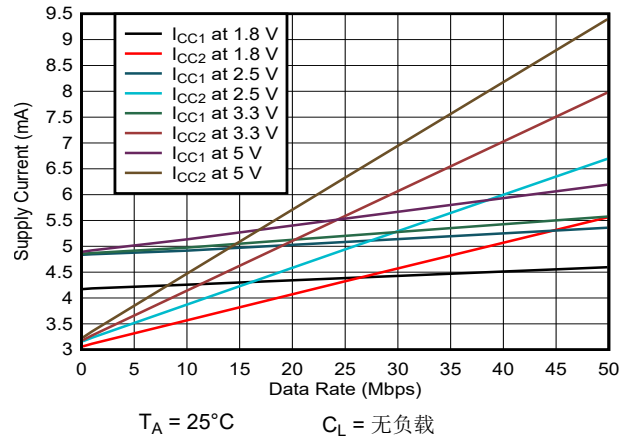
图 6-4. ISO6763 电源电流与数据速率间的关系 (无负载)
