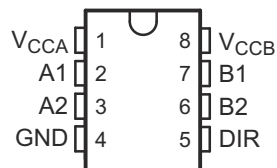
图 4-1. DCU 封装，5 引脚 VSSOP ( 顶视图 )
