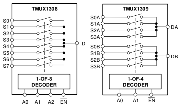
TMUX1308 和 TMUX1309 方框图
