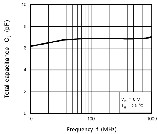
Fig. 8.4 C_t - f
