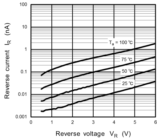
Fig. 8.2 I_R - V_R
