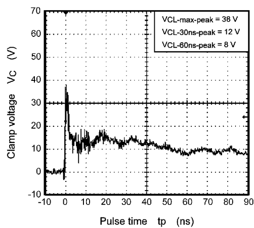
Fig. 5.1.1 +8 kV
