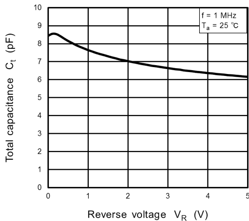
Fig. 8.3 C_t - V_R
