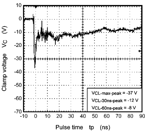
Fig. 5.1.2 -8 kV
