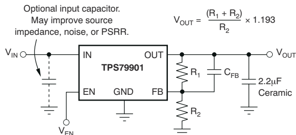
典型应用电路：可调电压版本
