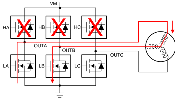
图 8-36. Brake State
