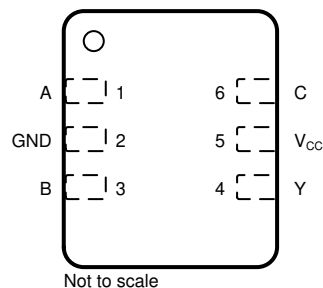
图 4-2. YZP 封装、6 引脚 DSBGA (底视图)
