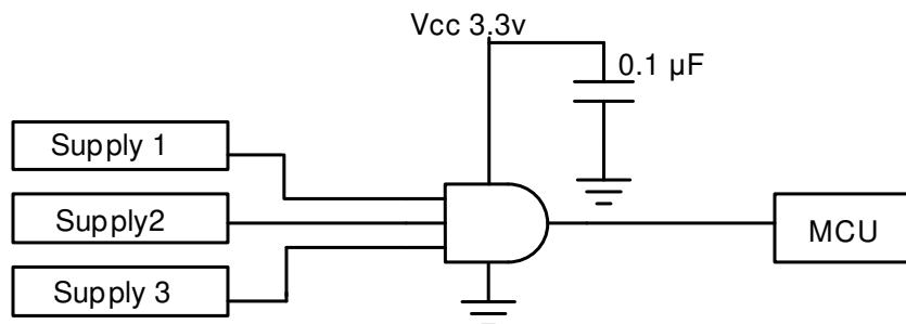
图 8-1. 典型应用图
