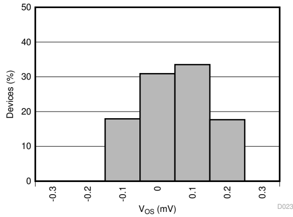
图 5-17. Offset Error Histogram
