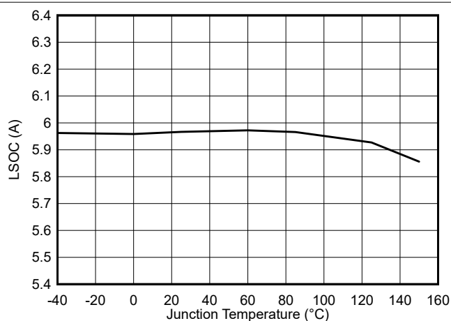
图 5-12. TPS54538 低侧电流限值与结温间的关系
