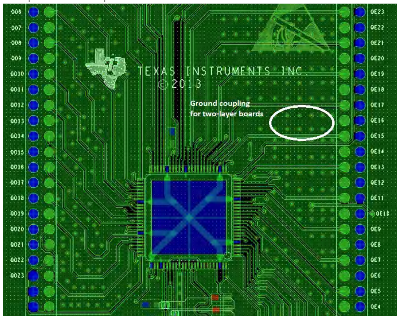
图 8-9. Data Route
