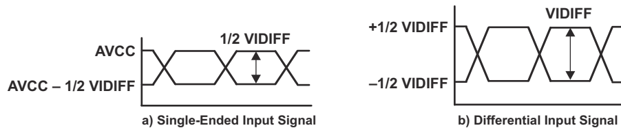
图 7-2. TMDS Inputs
