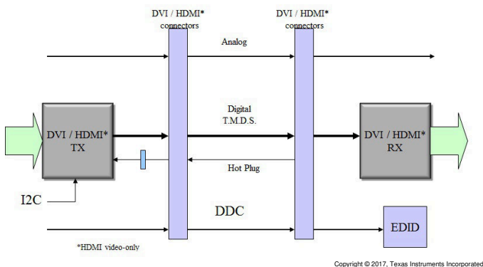
TFP401A-Q1 框图
