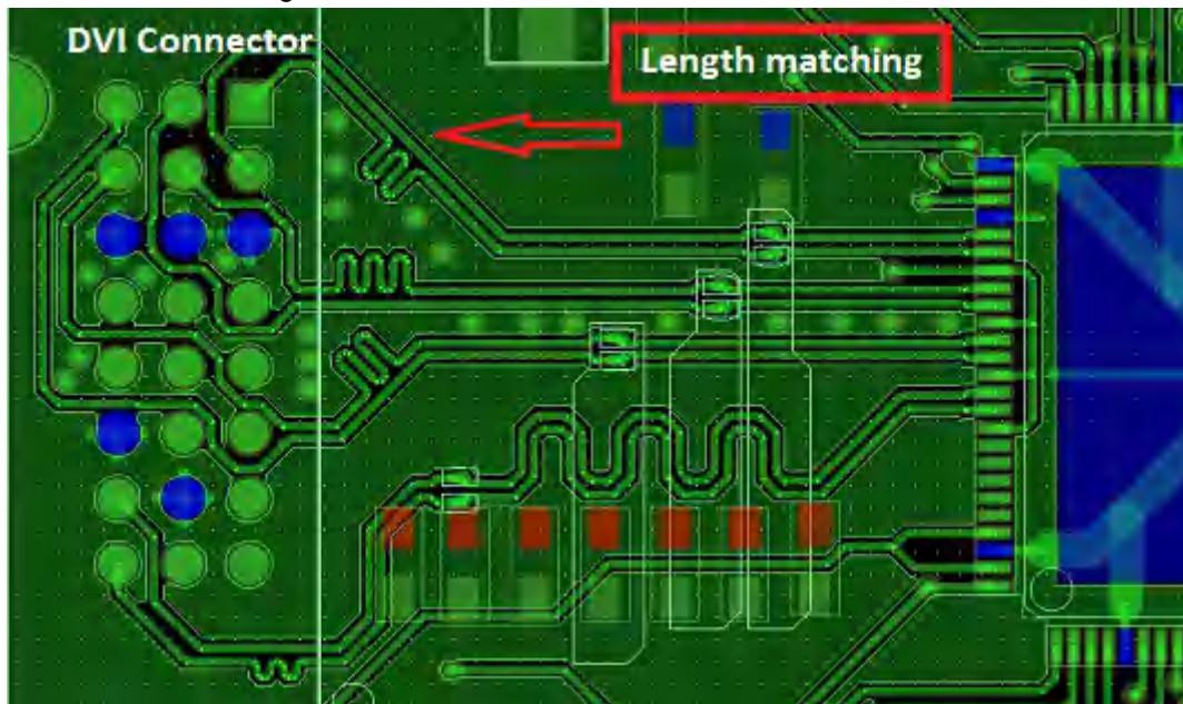
图 8-8. DVI Connector
