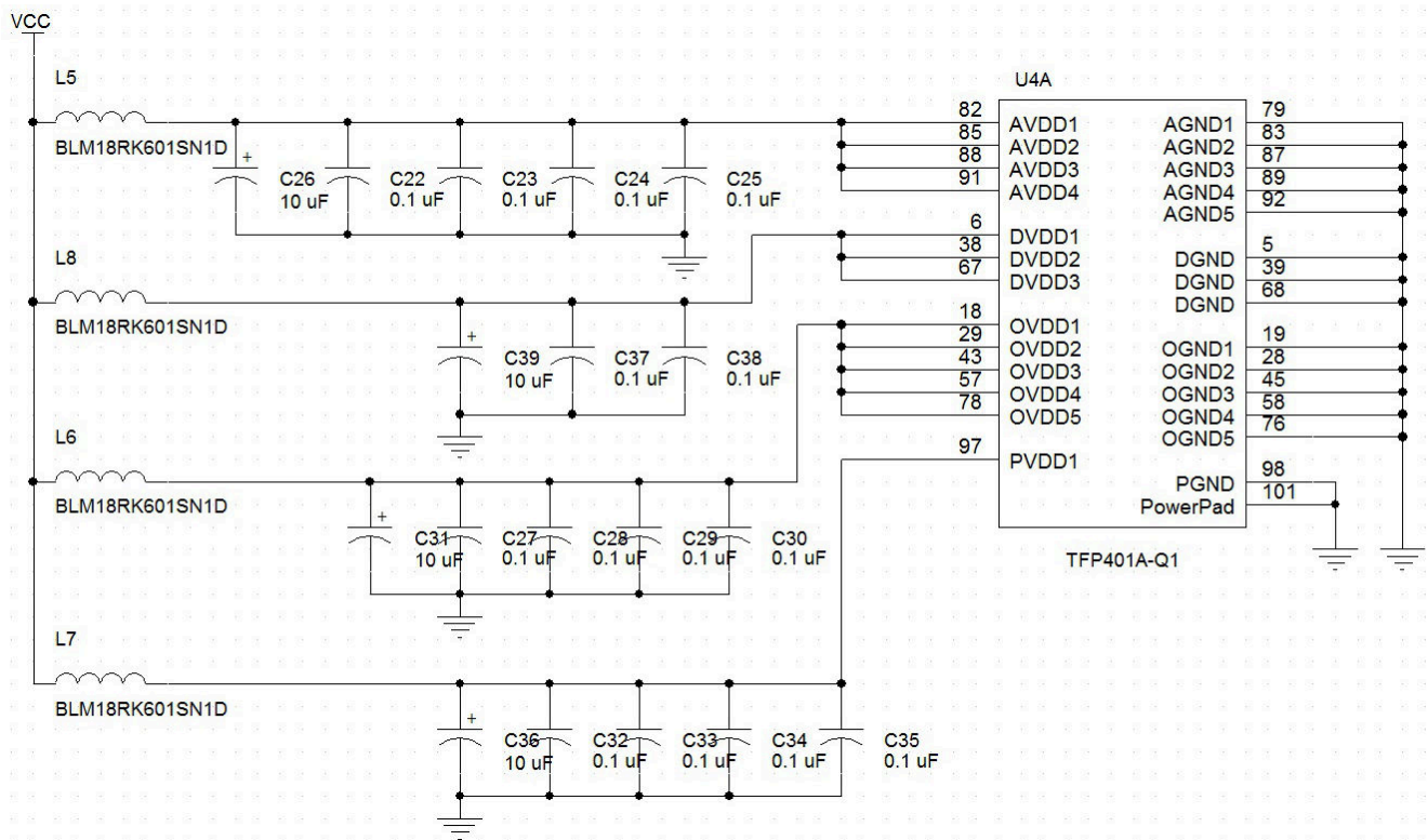
图 8-4. TFP401A-Q1 App Info Power Decoupling
