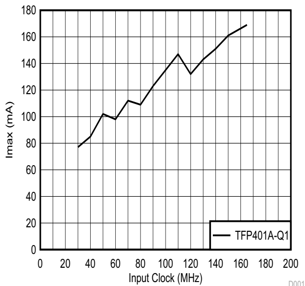
图 6-14. I_{max} vs Input Frequency
