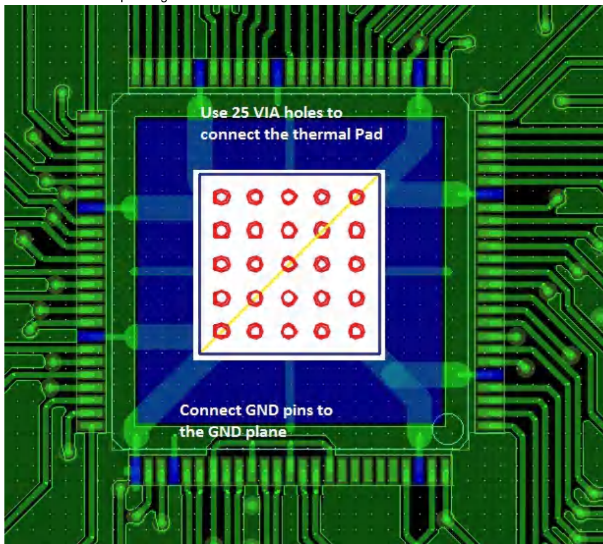
图 8-10. GND Route
