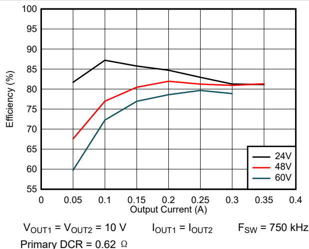
图 8-2. Efficiency
