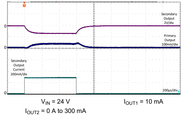
图 8-9. Load Transient on Secondary Output
