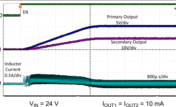
图 8-6. Light Load Start-Up from EN
