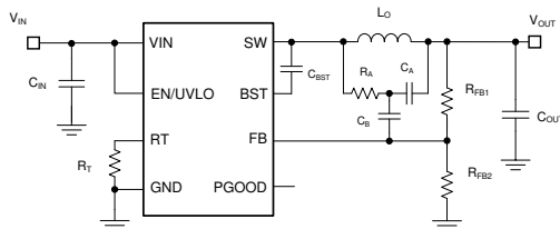
典型降压应用电路
