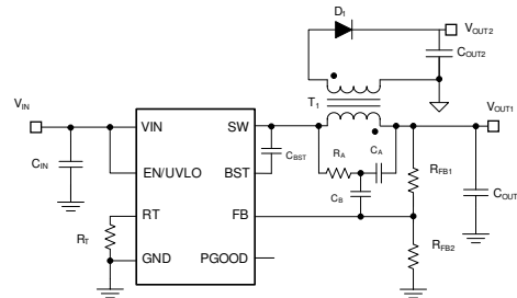
典型 Fly-Buck™ 转换器应用电路
