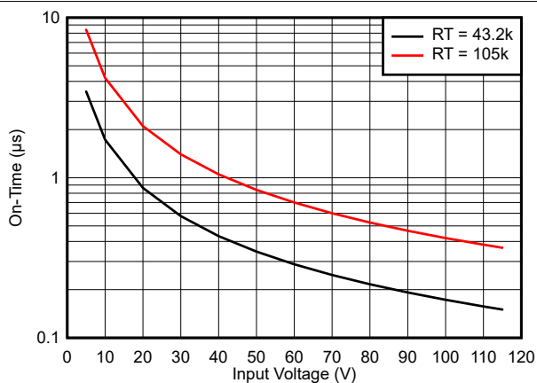
图 6-4. COT On Time Versus Input Voltage
