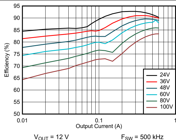
图 8-16. Efficiency: V_{OUT} = 12\text{ V}
