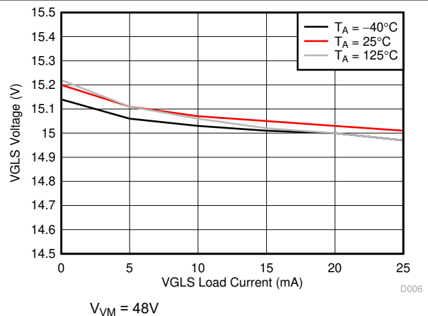
图 7-6. VGLS 电压与负载电流之间的关系
