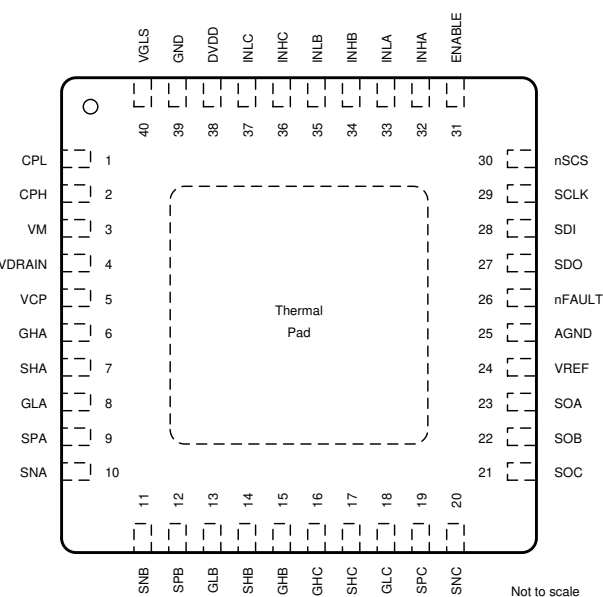
图 6-4. DRV8353FS RTA 封装 40 引脚 WQFN (带有外露散热焊盘) 顶视图
