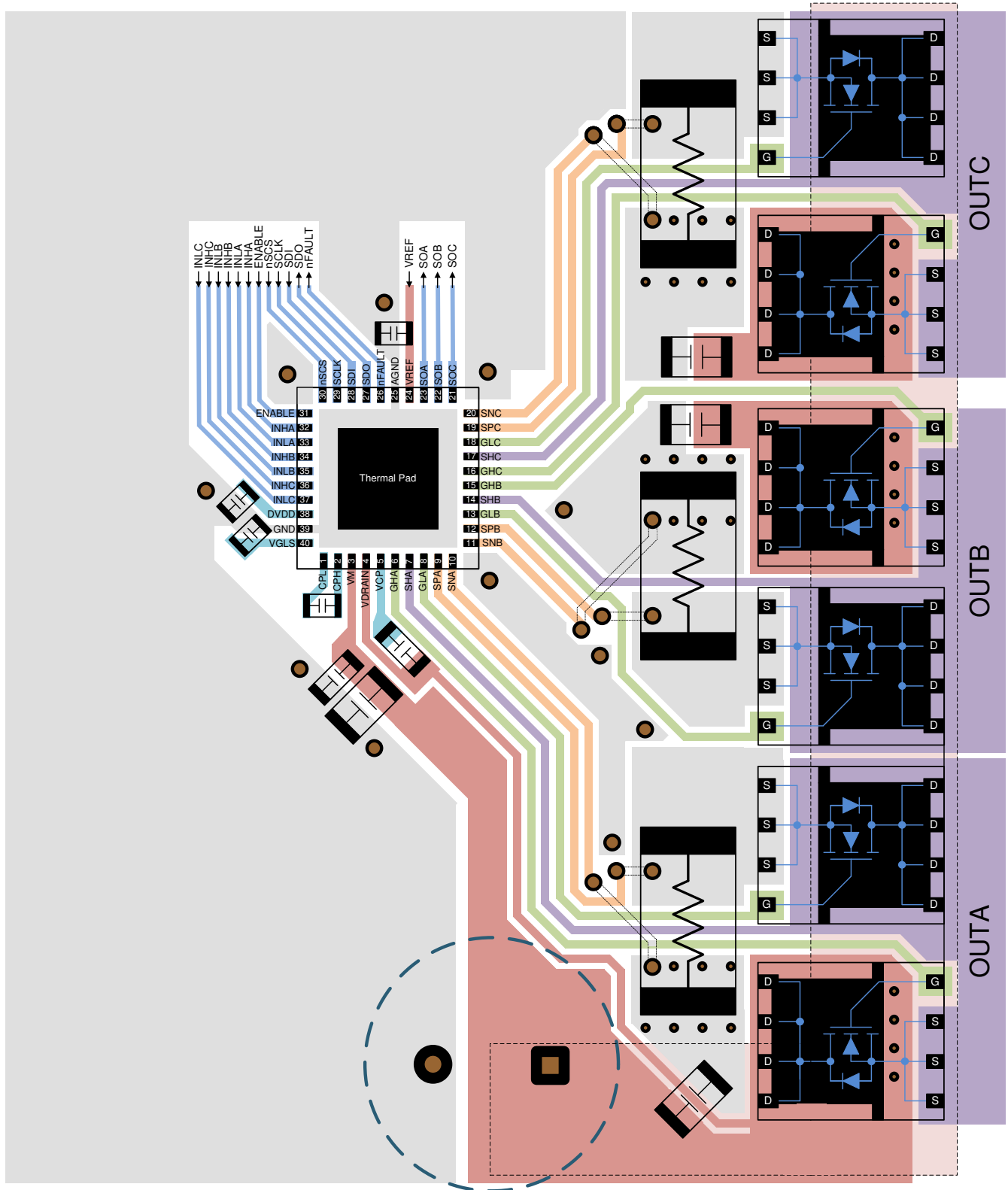
图 11-1. 布局示例
