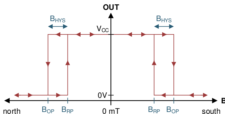
图 7-3. 全极功能
