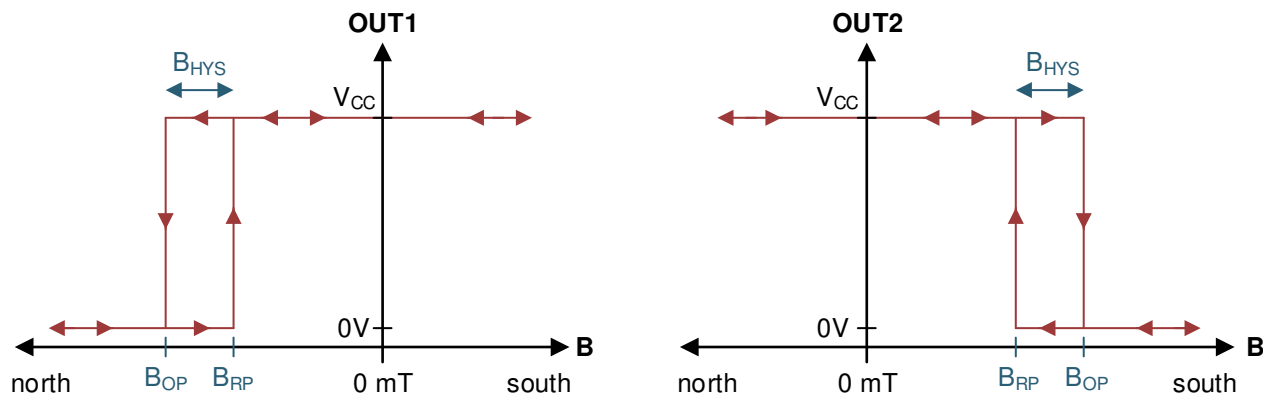
图 7-4. 单极功能
