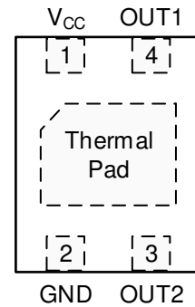
图 5-4. DU、DG、FD 版本 DMR 封装 4 引脚 X2SON 顶视图
